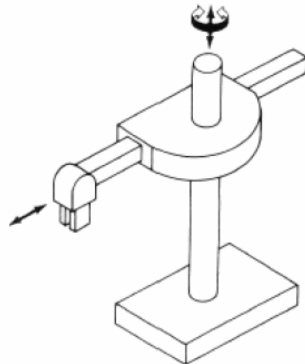
Cilíndrico
