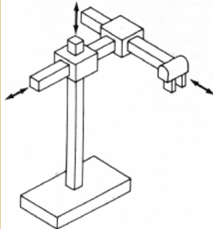
Cartesiano ou Retangular
