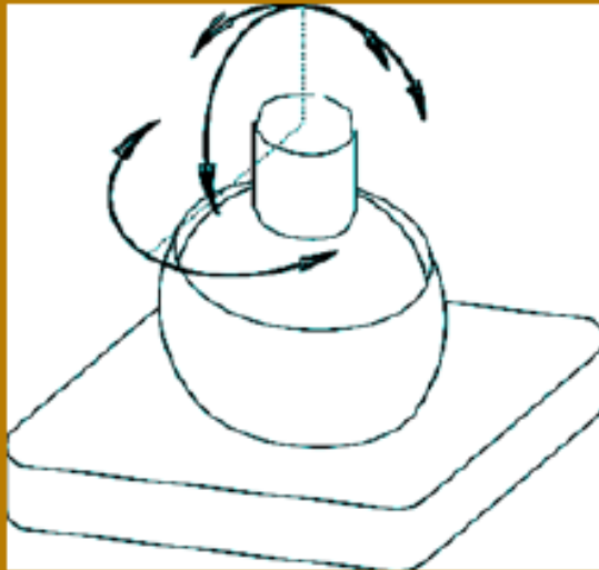
Junta Esférica (3 GDL)
