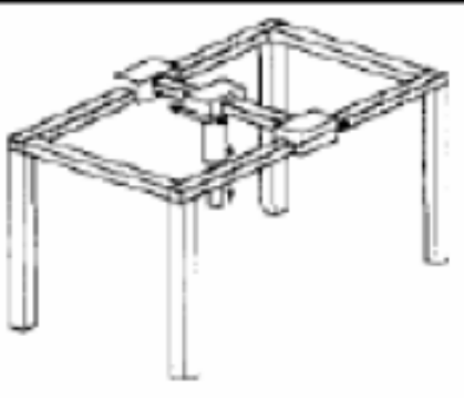
Robô Cartesiano
