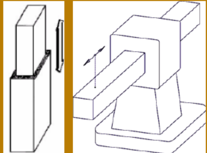
Junta Prismática (1 GDL)
